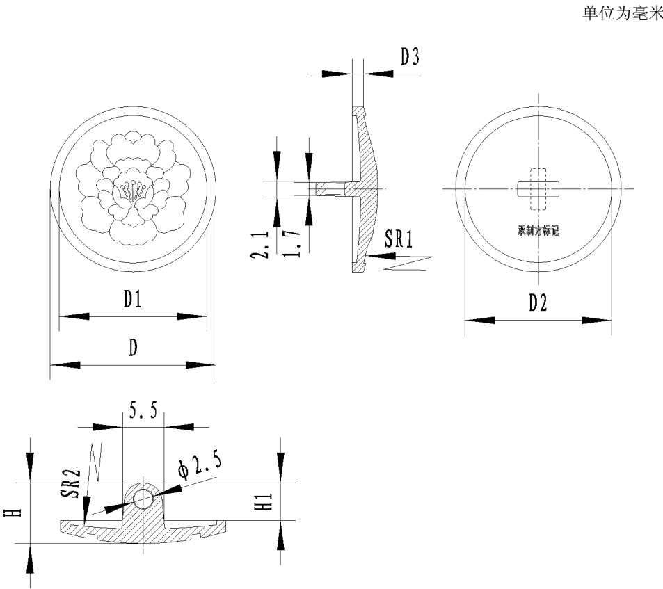
图 68 金属扣结构和主要尺寸
