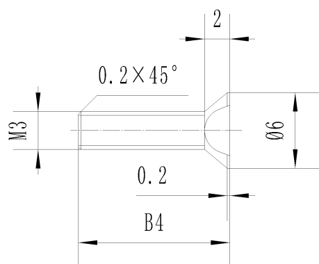
图 53b 螺钉结构及主要尺寸
