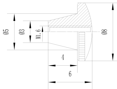
图 63c 螺母结构及主要尺寸
