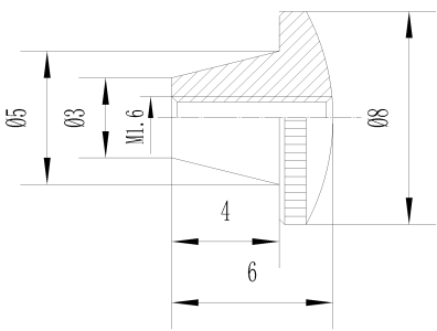
图 61c 螺母结构及主要尺寸
